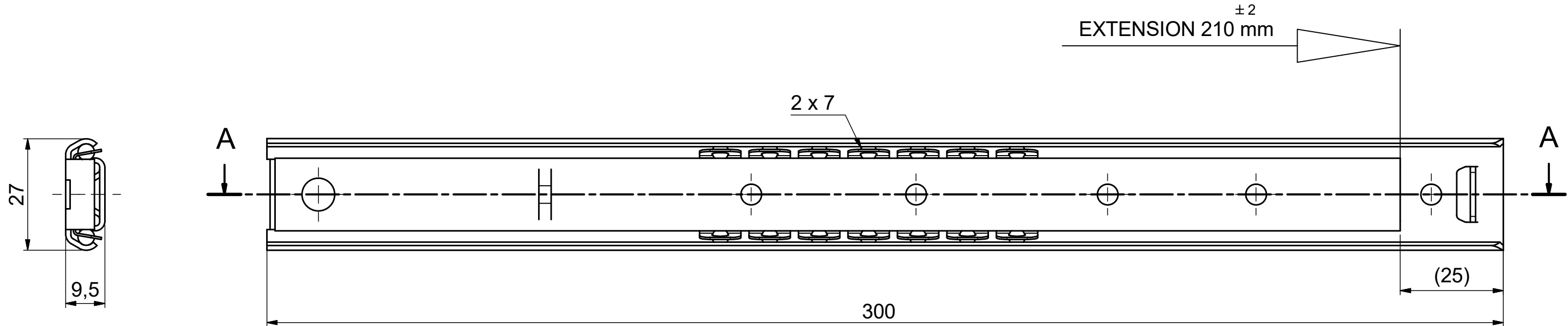
SECTION A-A
